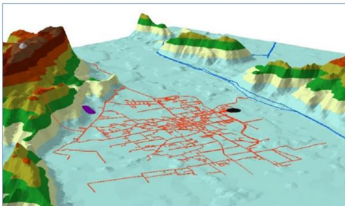
Figura 8. Ubicaciones alternativas para construcción Tanques Compensación. Alternativa 1 (Negro); Alternativa 2 (Azul).
